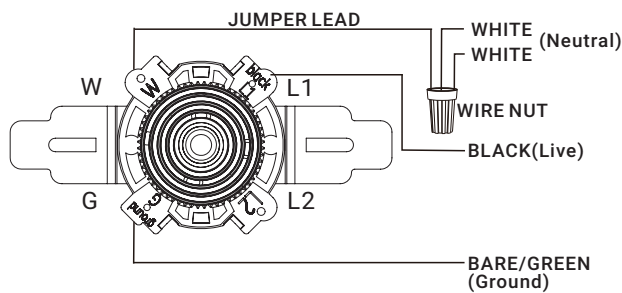
WIRING DIAGRAM#3:
