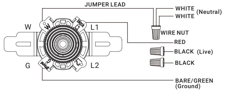
WIRING DIAGRAM#5:
