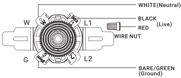
WIRING DIAGRAM#2:
