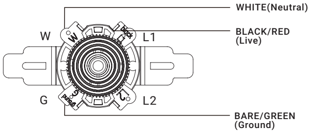
WIRING DIAGRAM#1:
