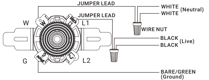
WIRING DIAGRAM#4:
