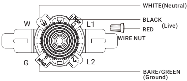
WIRING DIAGRAM#2:
