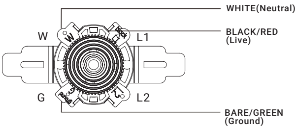
WIRING DIAGRAM#1:
