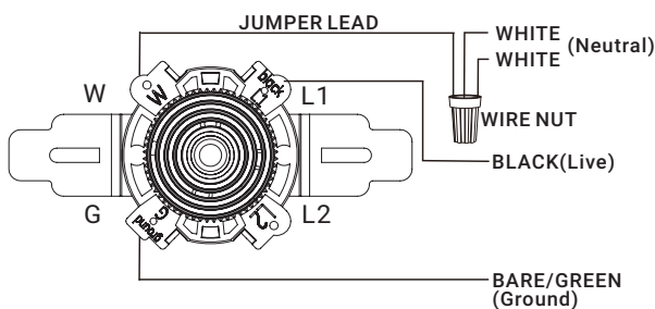
WIRING DIAGRAM#3:
