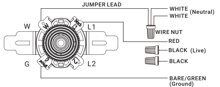
WIRING DIAGRAM#5:
