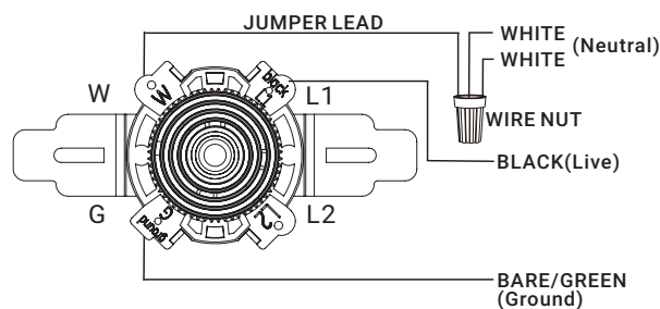
WIRING DIAGRAM#3:
