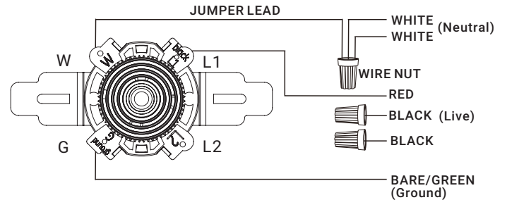
WIRING DIAGRAM#5:
