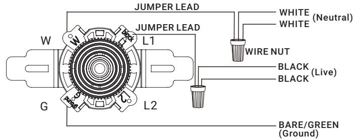
WIRING DIAGRAM#4:
