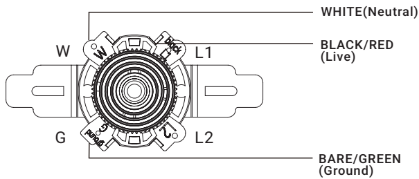
WIRING DIAGRAM#1:
