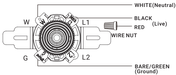
WIRING DIAGRAM#2:
